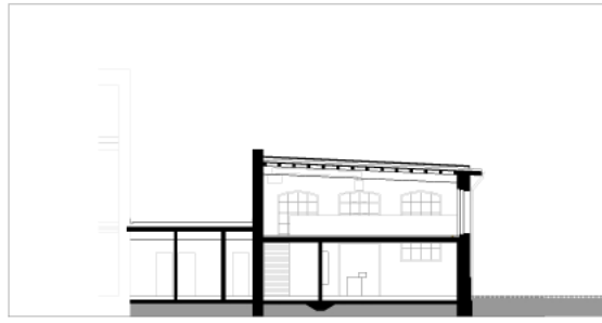
SCHNITT A-A
