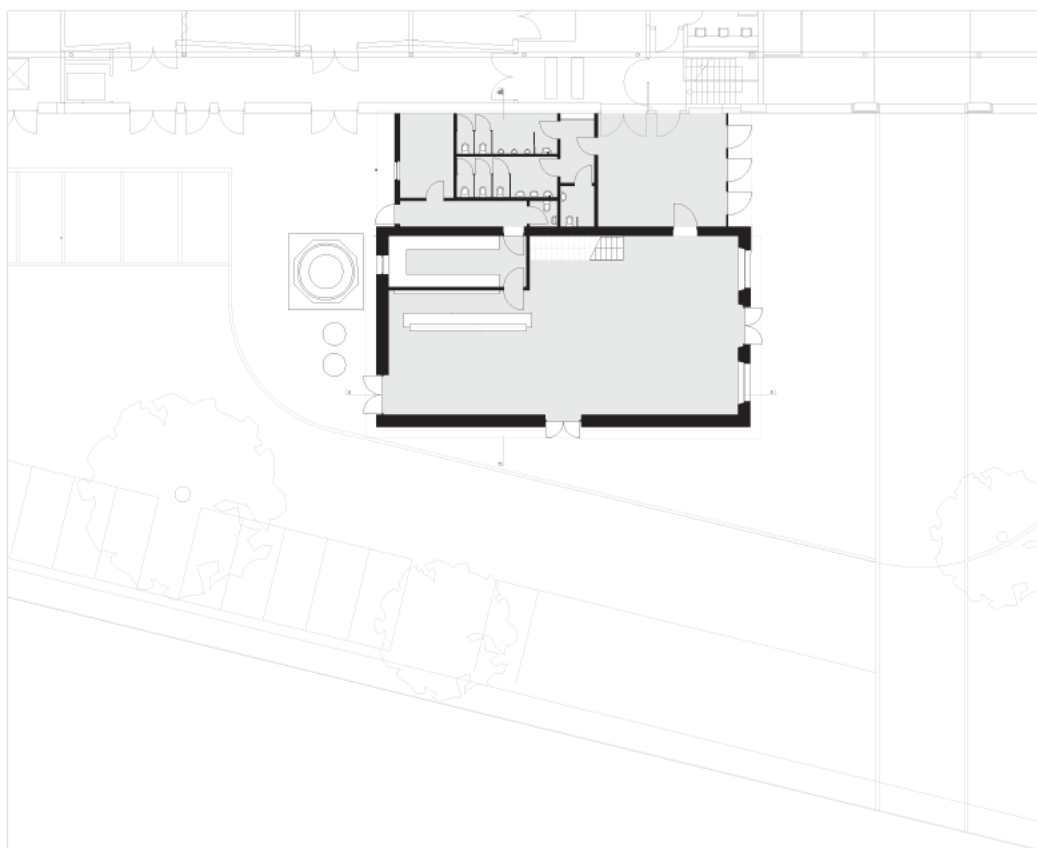
ERDGESCHOSS
